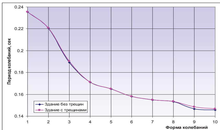
Рис. 12 – Периоды колебаний по первым 10-ти формам для здания с трещинами и без трещин
