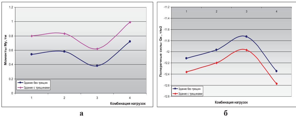
Рис. 11 – Моменты M_y (а), тм, и поперечные силы Q_x (б) в стене пристройки Н – А по оси 9 в зданиях с трещинами и без трещин
