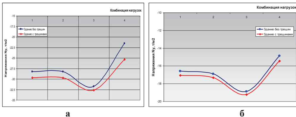
Рис. 9 – Напряжения N_y , т/м 2 , в стене фасада пристройки: а) по оси 9; б) по оси 13
